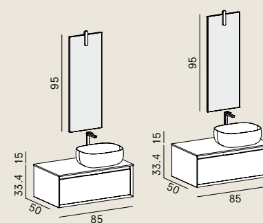
Materia Vip 03 L 85.6 × P 50.5 cm p — 22 WL verde comodoro velvet / 901L0 bianco lucido
