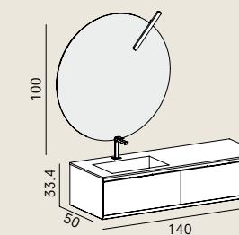
Materia Vip 06 L 140.6 × P 50.5 cm p — 34 (L 155 cm con sporg. specchio) 905V0 bianco velvet / 7A2 noce antico biondo
