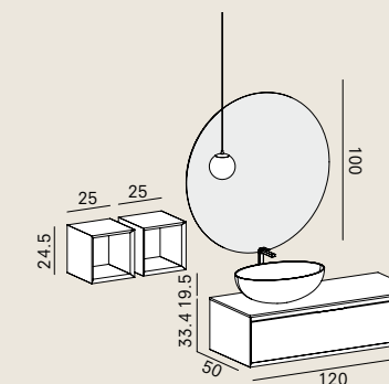
Materia Vip 02 L 120.6 × P 50.5 cm p — 16 (L 140 cm con sporg. specchio) WJ grigio Londra velvet / 8AA rovere antico inchiostro
