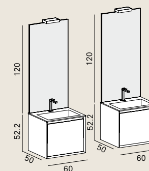
Materia Vip 08 L 60.6 × P 50.5 cm p — 48 905V0 bianco velvet / 7A1 noce antico scuro
