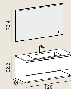
Materia Vip 01 L 120.6 cm × P 50.0 cm p — 04 905V0 bianco velvet / 8A2 rovere antico crema
