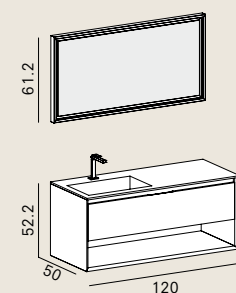
Materia Vip 07 L 120.6 × P 50.5 cm p — 42 WO grigio bromo velvet / 8A8 rovere antico essenza
